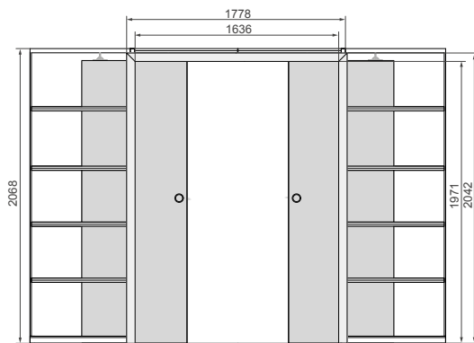
Kazeta dvojita G/K, dveřní křídlo / Kazeta dvojité G/K, dverné křídlo
