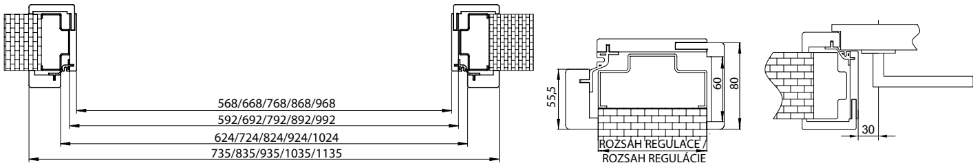
spojení zárubně / spojenie zárubne: 45°
