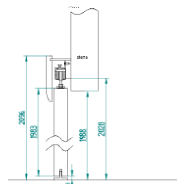
Nástenný posuvný nevstavaný systém
