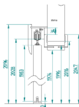
Nástenný posuvný vstavaný systém
